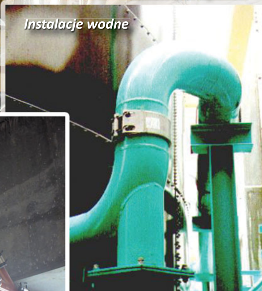
Systemy okrętowe
